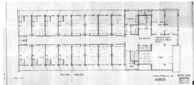
Plànols de la Clínica Meritxell de l'arquitecte Josep Canela i Tomàs. Fons Enric Dilme
